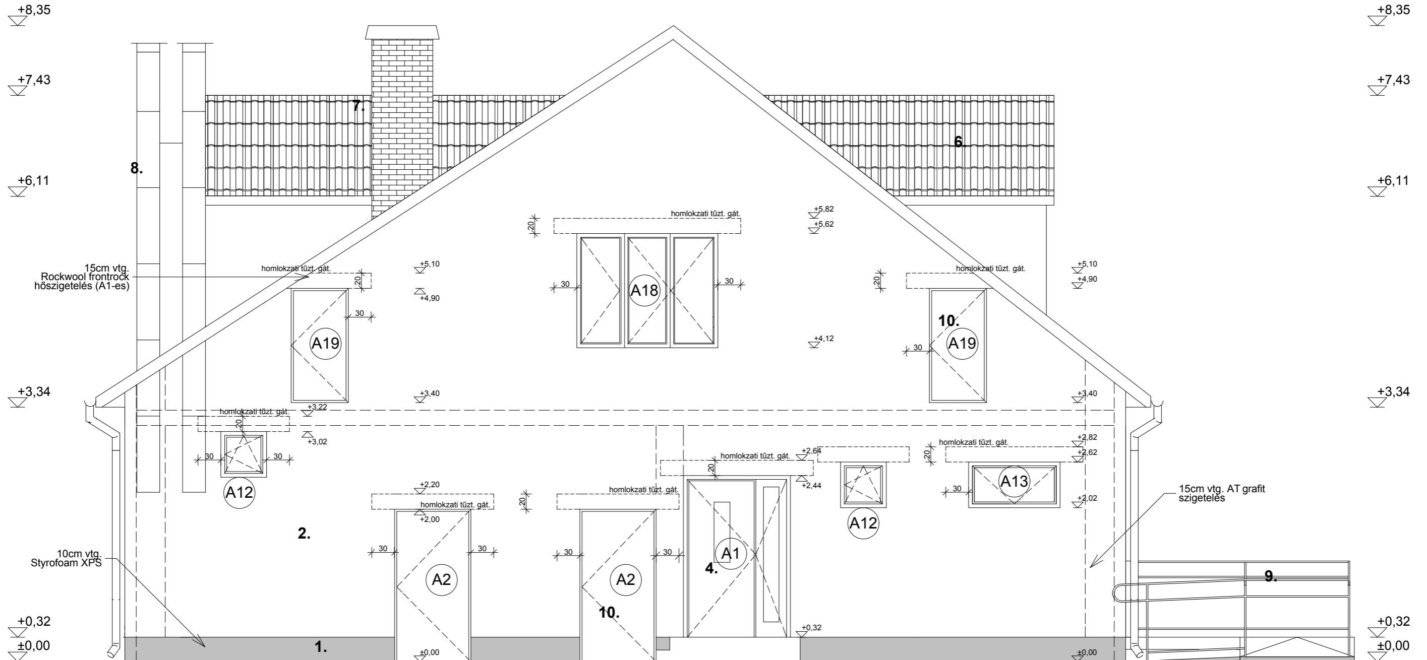
nyugati homlokzat, m=1:50
