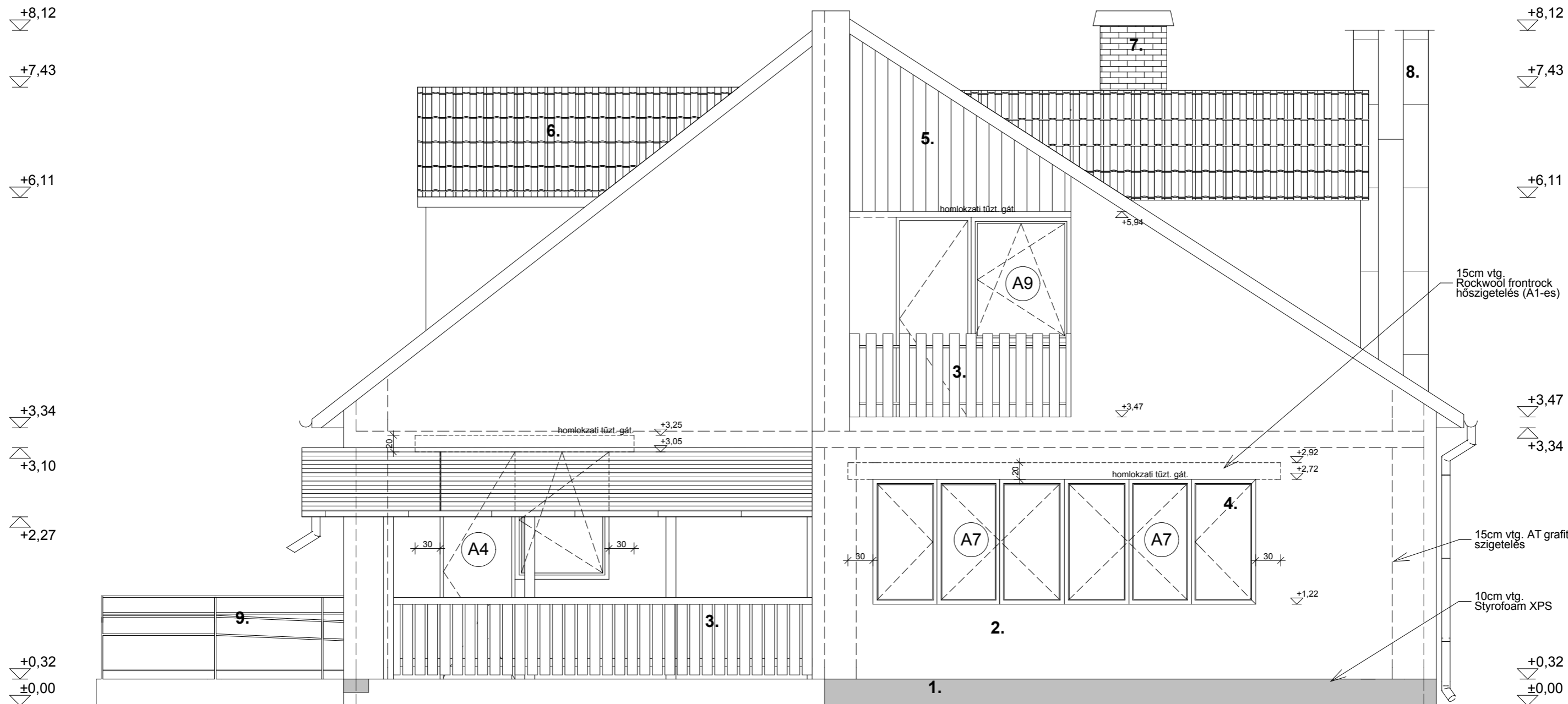
keleti homlokzat, m=1:50
