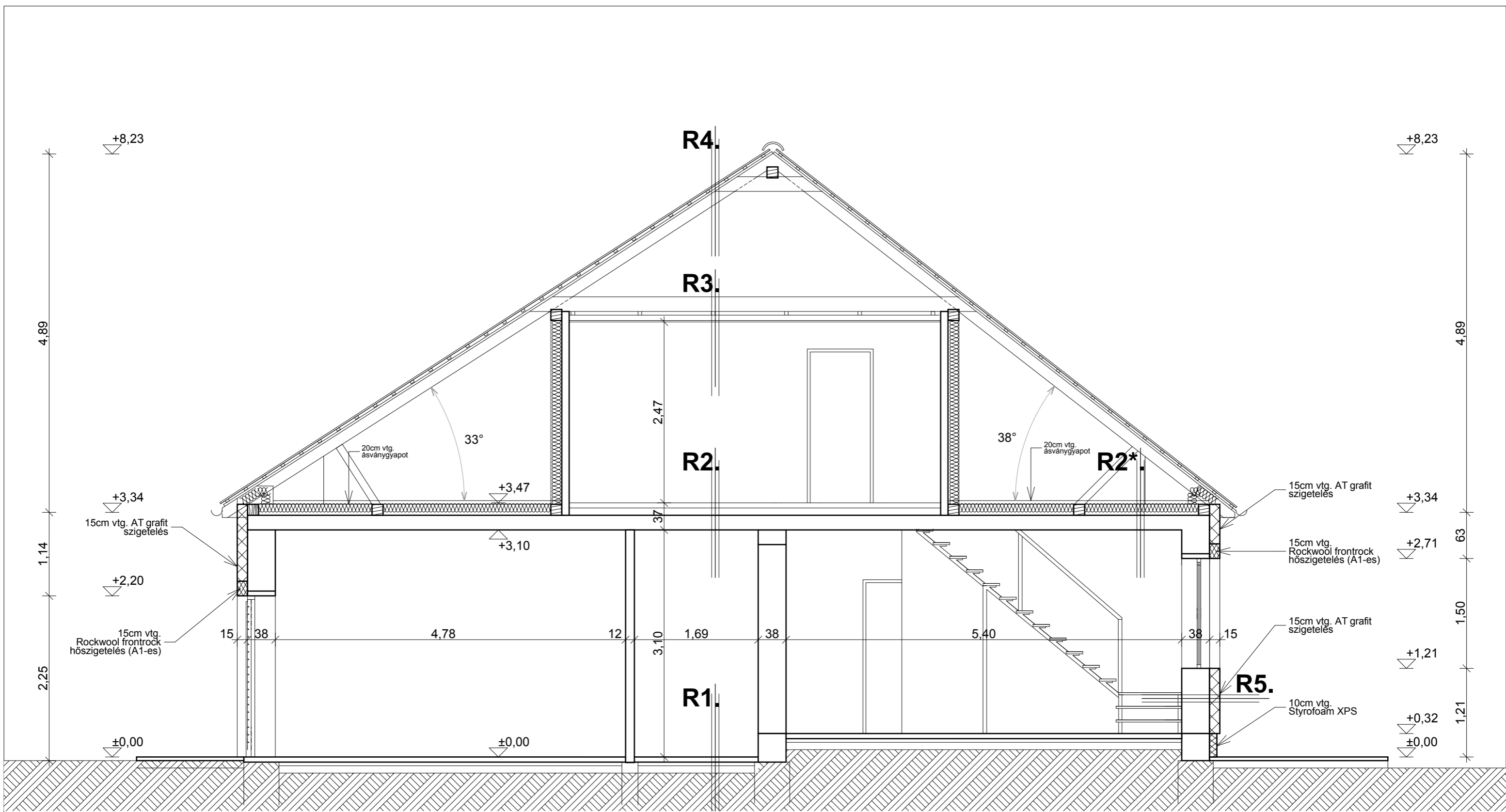
a-a metszet m=1:50
