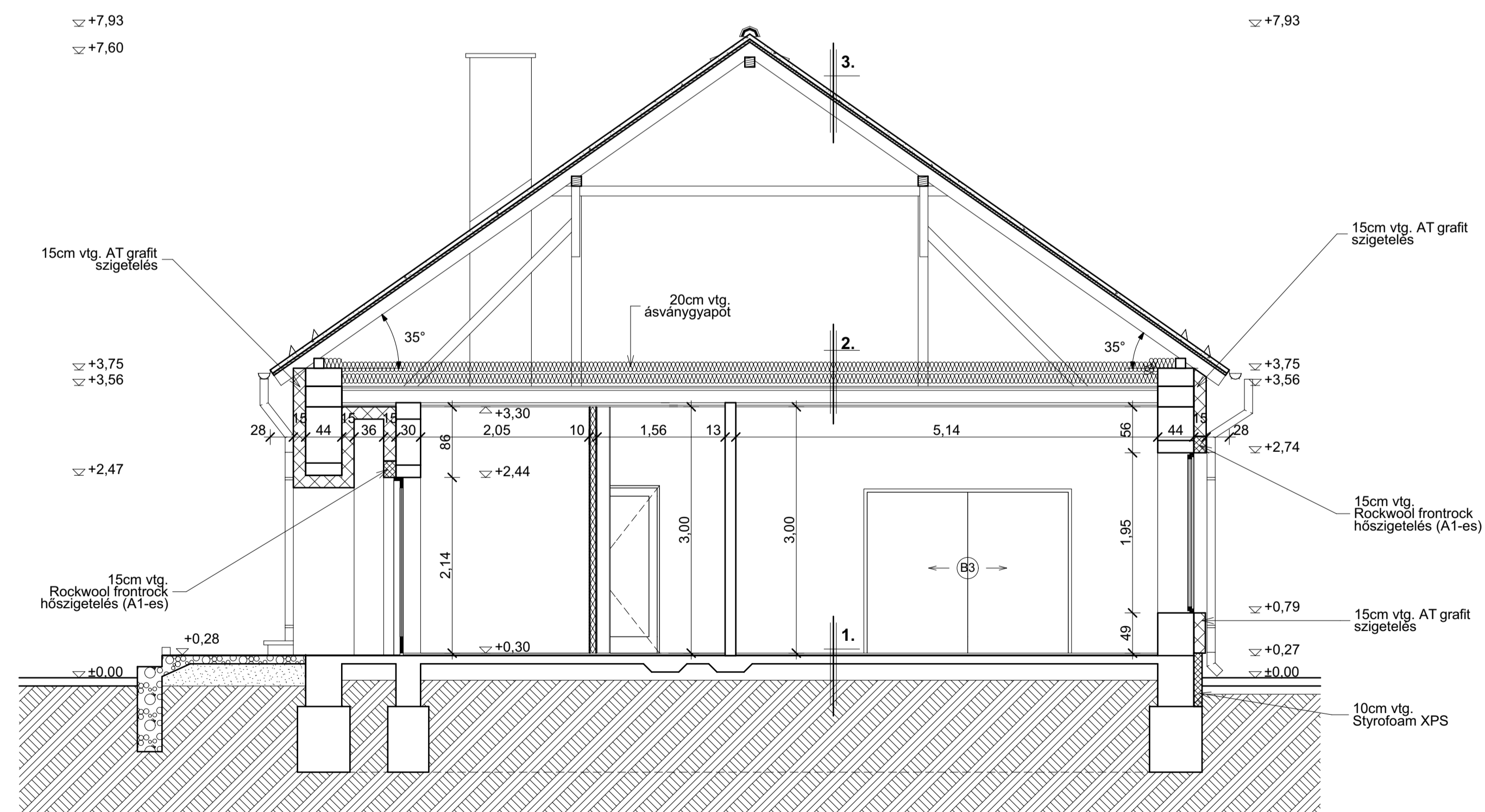
B-B metszet, m=1:50
