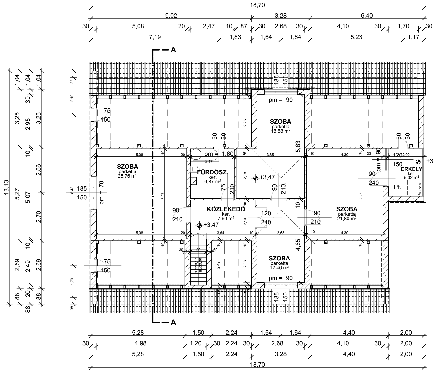
tetőtéri alaprajz m=1:100 nettó alapterület: 93,36m 2
