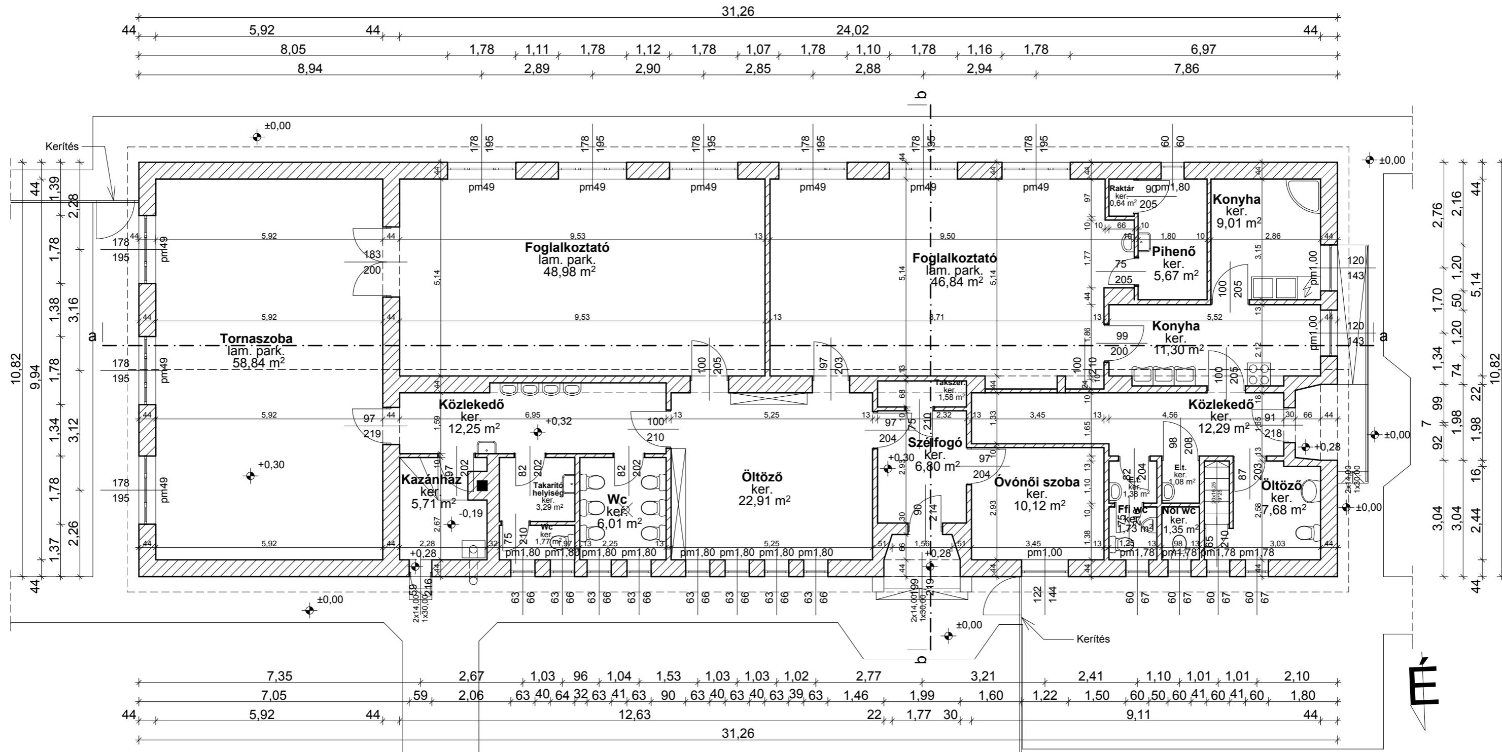
alaprész, m=1:100 nettó alapterület: 277,53 m 2
